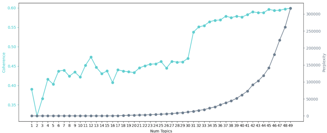
図 13：バイデン氏のツイートの Coherence と Perplexity、トピック数のグラフ
