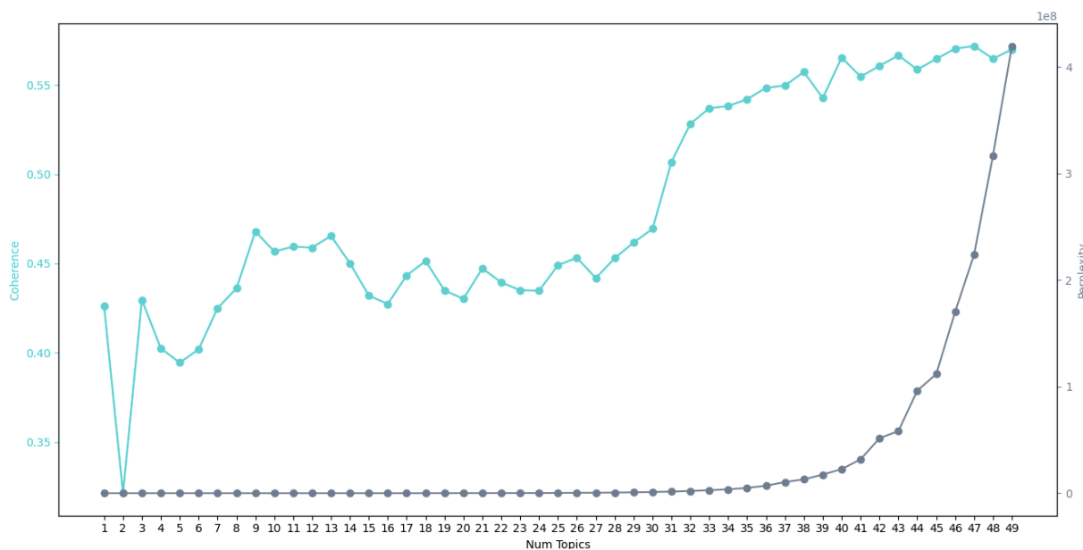
図 11：トランプ氏のツイートの Coherence と Perplexity、トピック数のグラフ
