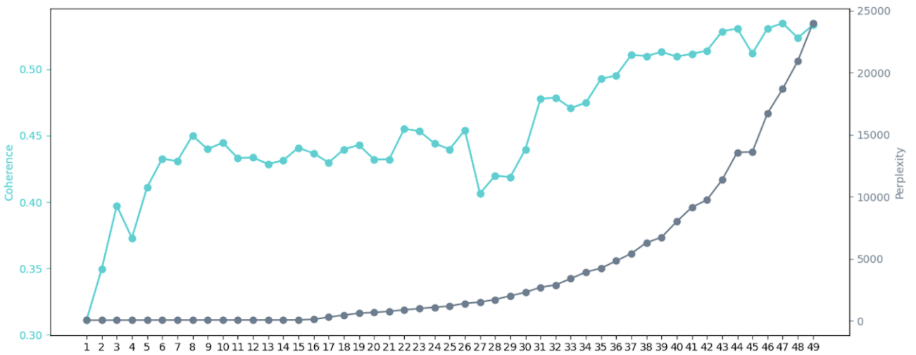
図 14：ハリス氏のツイートの Coherence と Perplexity、トピック数のグラフ
