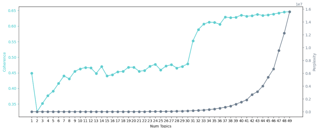
図 12：ペンス氏のツイートの Coherence と Perplexity、トピック数のグラフ
